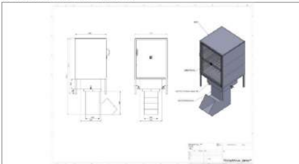
Gambar 2. Wireframe Rancangan Kompor Biomassa IoT
